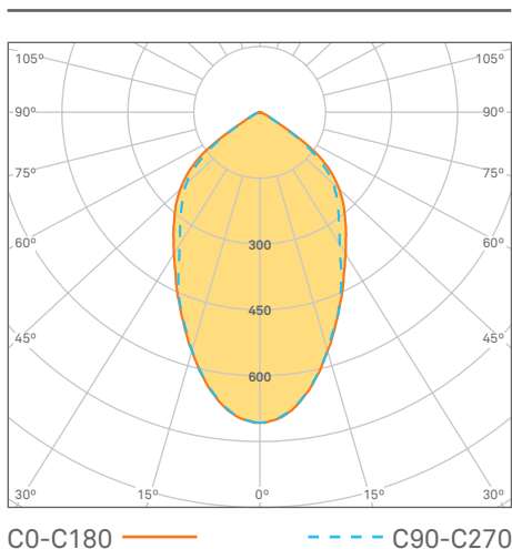
60 – Optik mit Abstrahlwinkel 60° Auf Anfrage erhältlich
