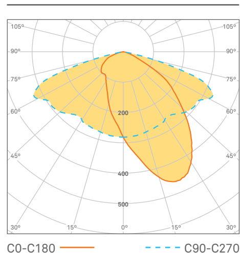
AS – asymmetrische Optik 90° Auf Anfrage erhältlich
