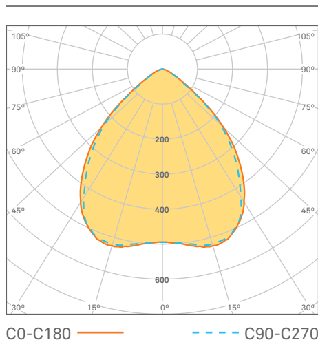
90 – Optik mit Abstrahlwinkel 90° Als Standard
