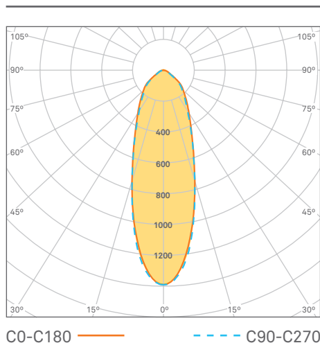
30 – Optik mit Abstrahlwinkel 30° Auf Anfrage erhältlich
